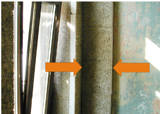
Dämmung einbindender Innenwände und Massivdecken mit einer 40 cm breiten Dämmschürze
